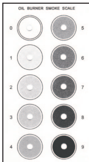
ESCALA DE COMPARAÇÃO ÍNDICE DE FULIGEM
